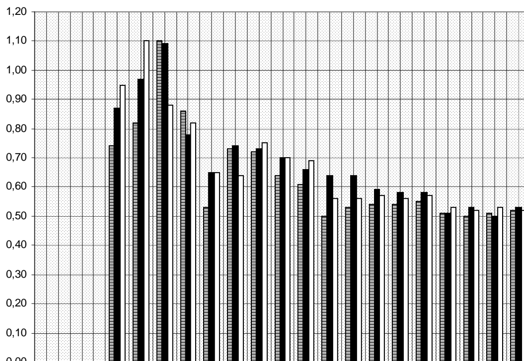
POHLTIVOST ALFA - DRÁŽKOVANÉ PANELE tl.16mm, 600x1000,2000; 300x2000mm AVS 1 32/3 - drážky osově 32mm ; křivka 1, 2, 3 dle distance D(cm), t (cm) tlumící vložky a hustotu a velikost děrování na rubové straně
