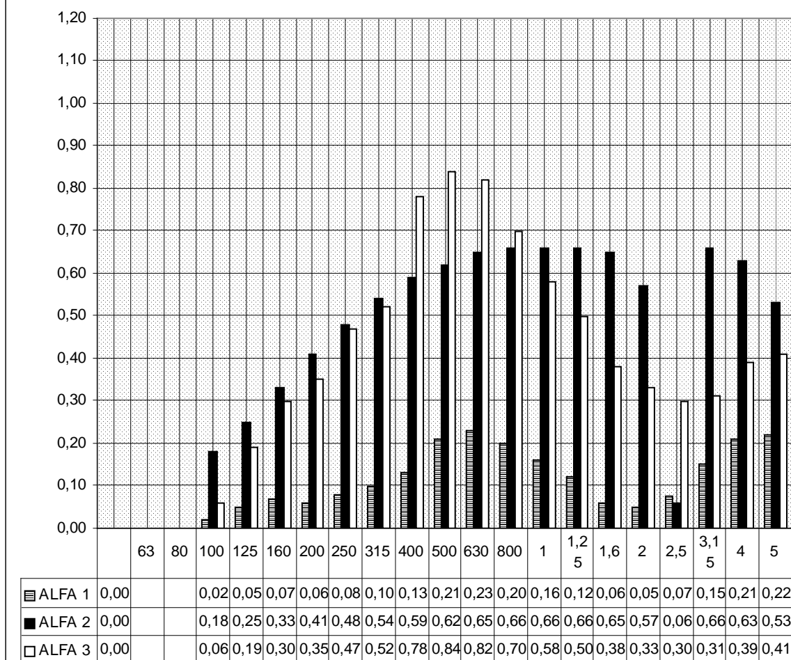
POHLTIVOST ALFA - PERFOROVANÉ KAZETY 600x600mm; tl. 12mm AVS 02 16/8 ; křivka 1, 2, 3 dle distance D(cm), t (cm) tlumící vložky
