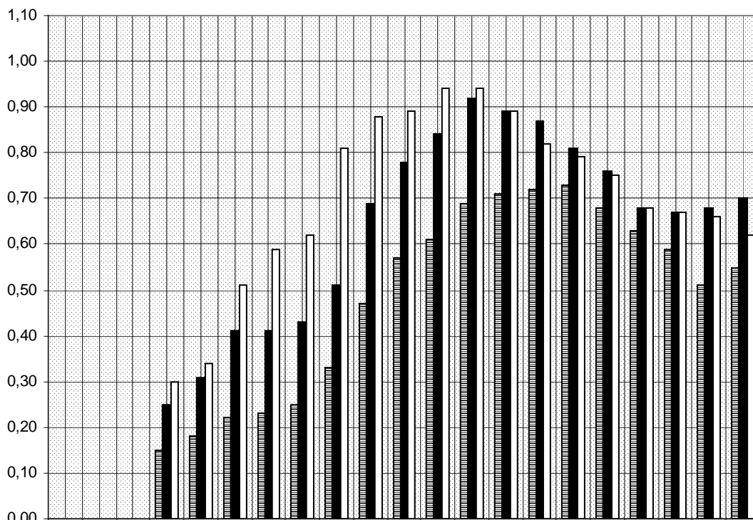
POHLTIVOST ALFA - DRÁŽKOVANÉ PANELY tl. 16mm, 600x1000,2000; 300x2000 AVS 2 16/3 - drážky osově 16mm ; křivka 1, 2, 3 dle distance D(cm), t (cm) tlumící v ložky a hustoty a velikost děrování na rubové straně
