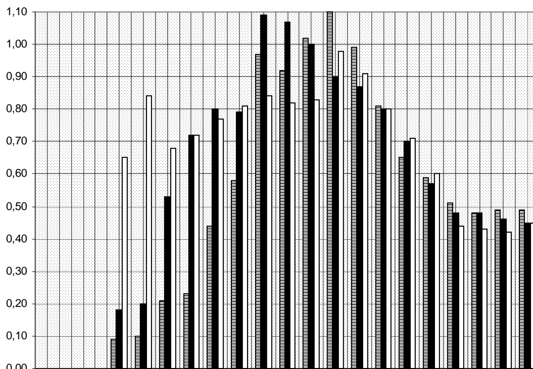
POHLTIVOST ALFA - DRÁŽKOVANÉ PANELE tl. 16mm, 600x1000,2000; 300x2000 AVS 3 8/3 - drážky osově 8mm ; křivka 1, 2, 3 dle distance D(cm), t (cm) tlumící vložky a hustotu a velikost děrování na rubové straně
