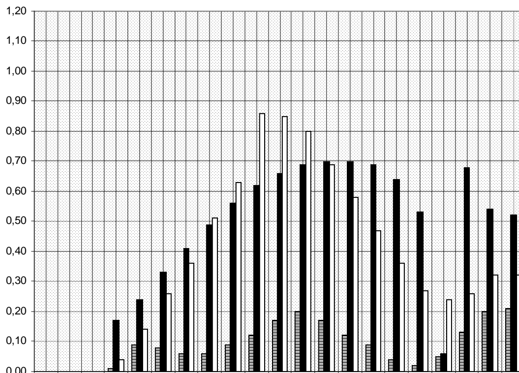
POHLTIVOST ALFA - PERFOROVANÉ KAZETY 600x600mm; tl. 12mm AVS 01 32/10 - oválné otvory ; křivka 1, 2, 3 dle distance D(cm), t (cm) tlumící vložky
